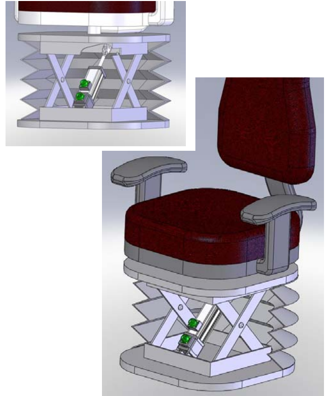
Tritex Actuator
